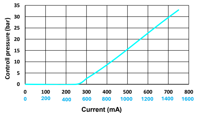
P-I CURVE (24 V_8,15 \Omega / 24 V_20,8 \Omega )
