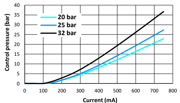
P-I CURVE (24 V)
